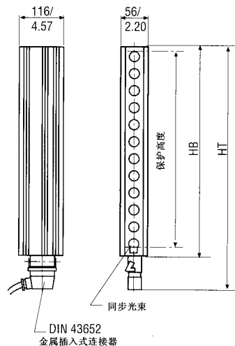
DIN43652 标准的金属连接器
